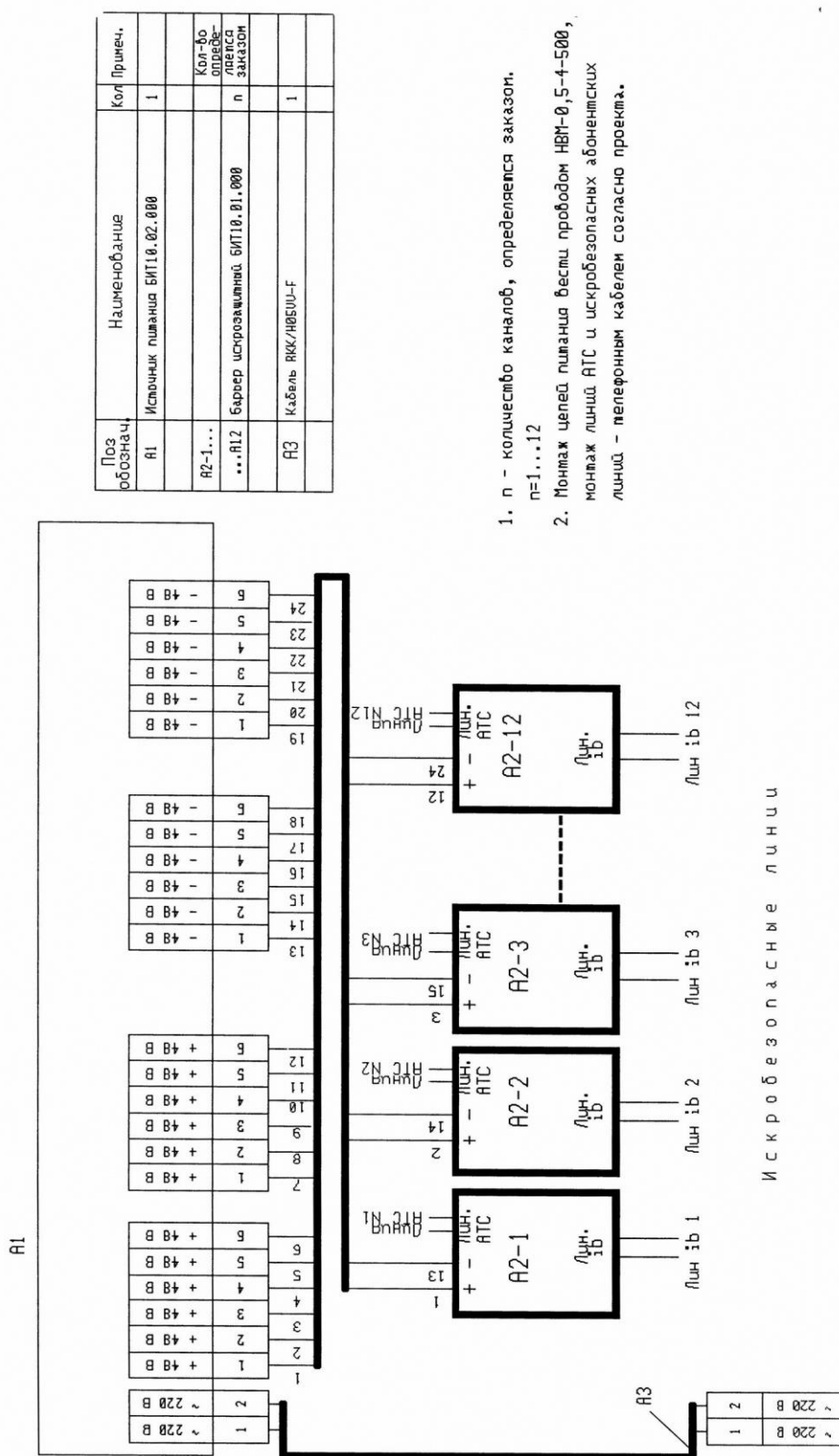
Схема электрическая подключений БИТ10.00.000-01 Э5.
