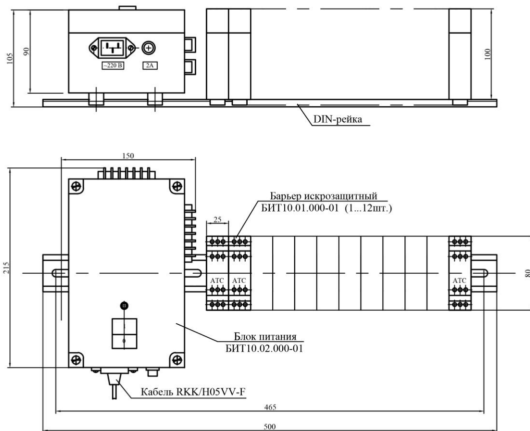
Сборочный чертеж БИТ10.00.000-01 СБ.
