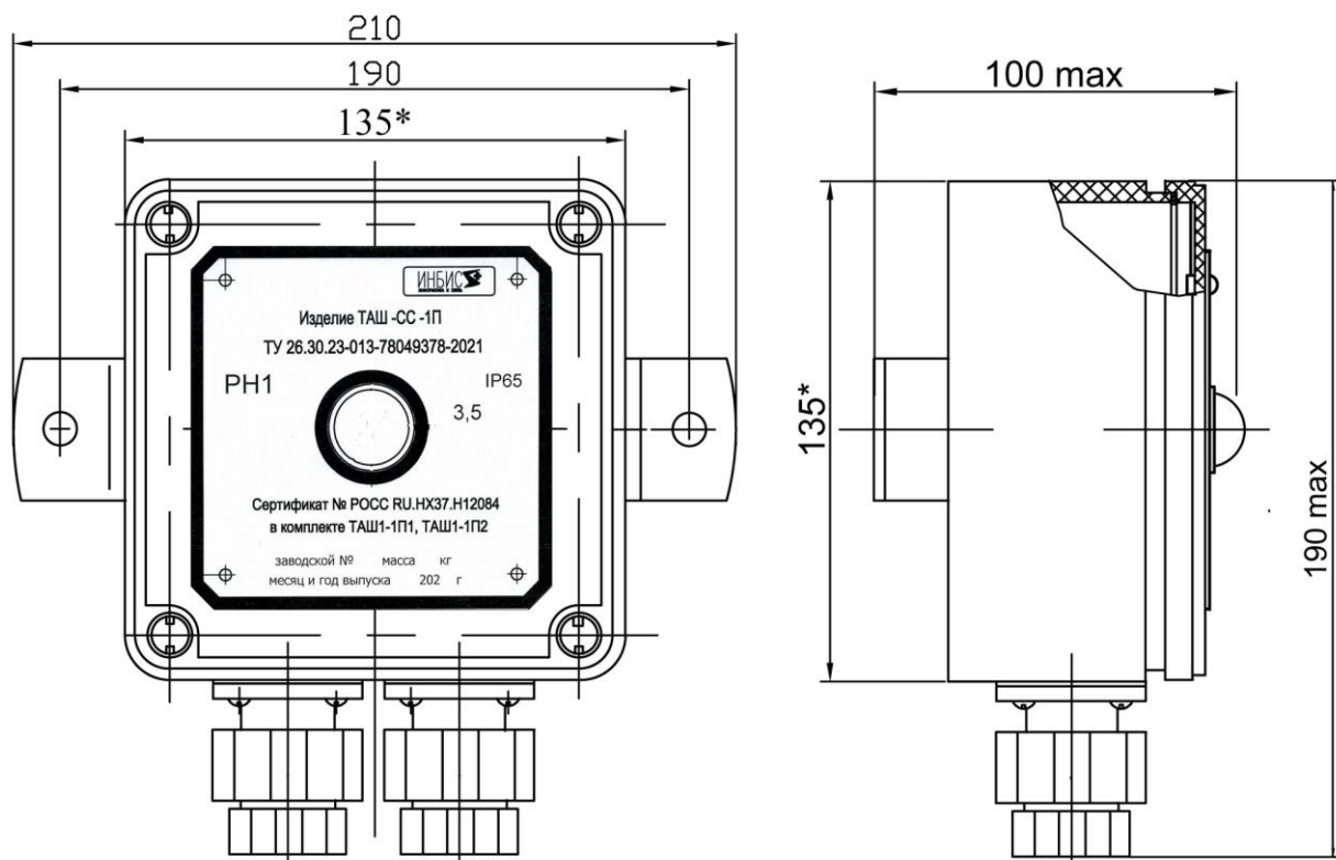
Сборочный чертеж устройства ТАШ-СС-1П
